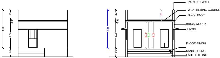
ELEVATION
