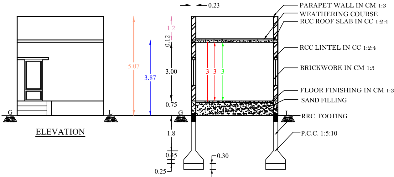
SECTION - AB
