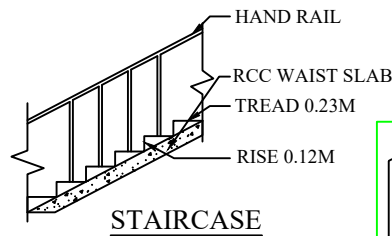
SECTION - AB
