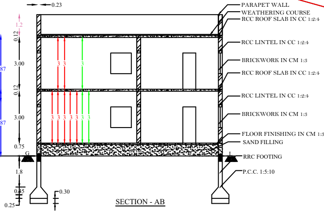
SECTION - AB
