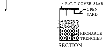
SECTION PLAN R.W.H
