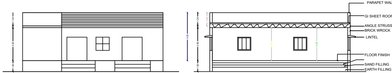
ELEVATION
