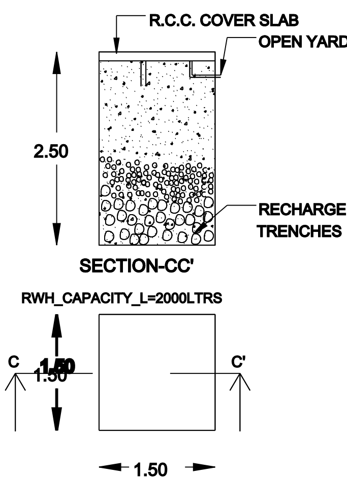
R.W.H
