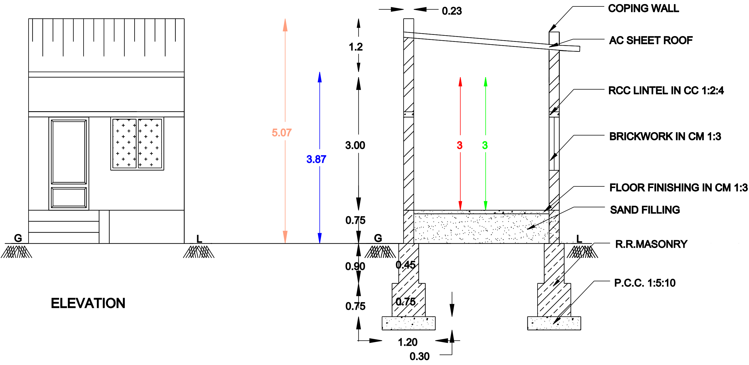
SECTION - AB
