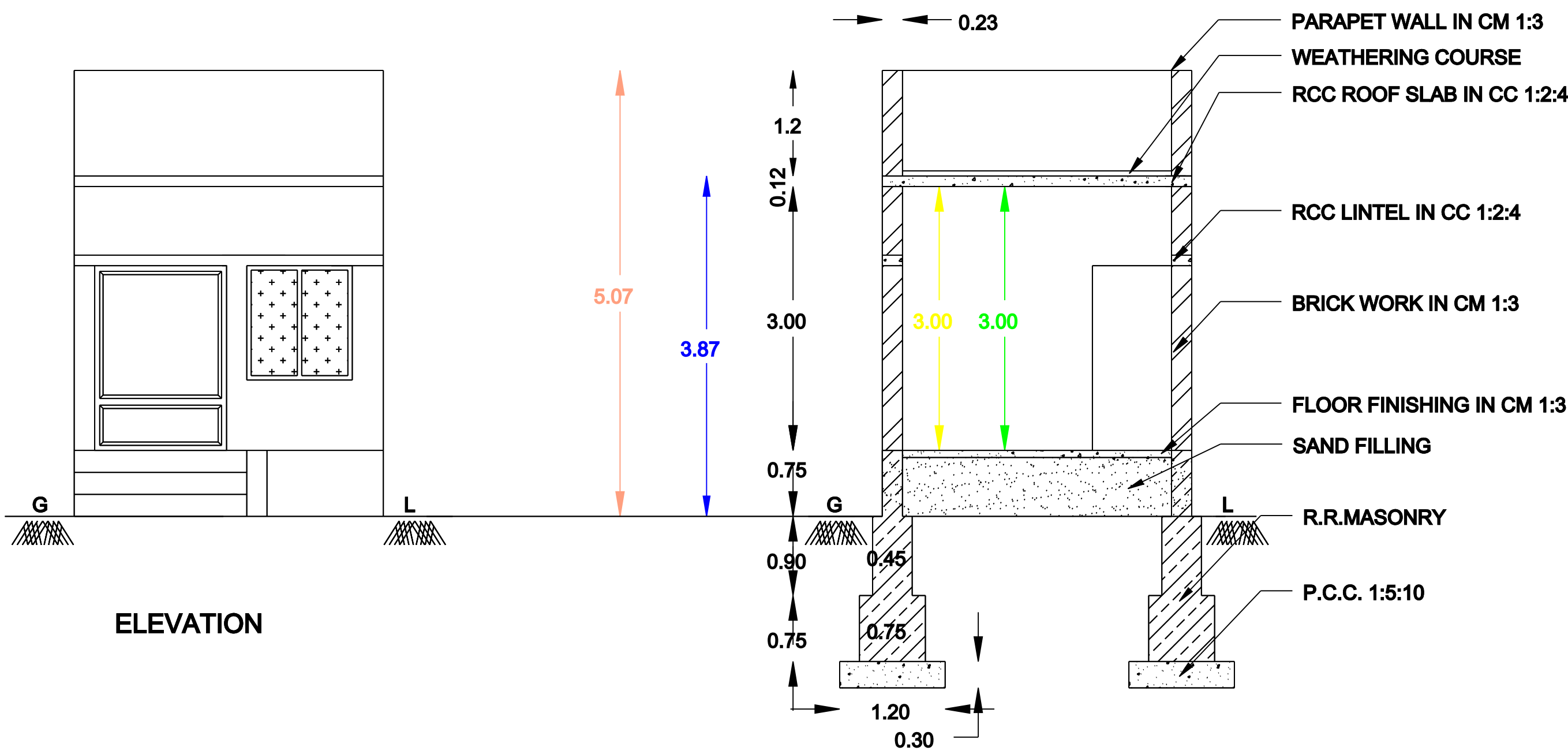
SECTION - AB
