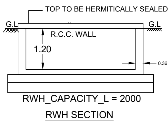
R.W.H. SECTION
