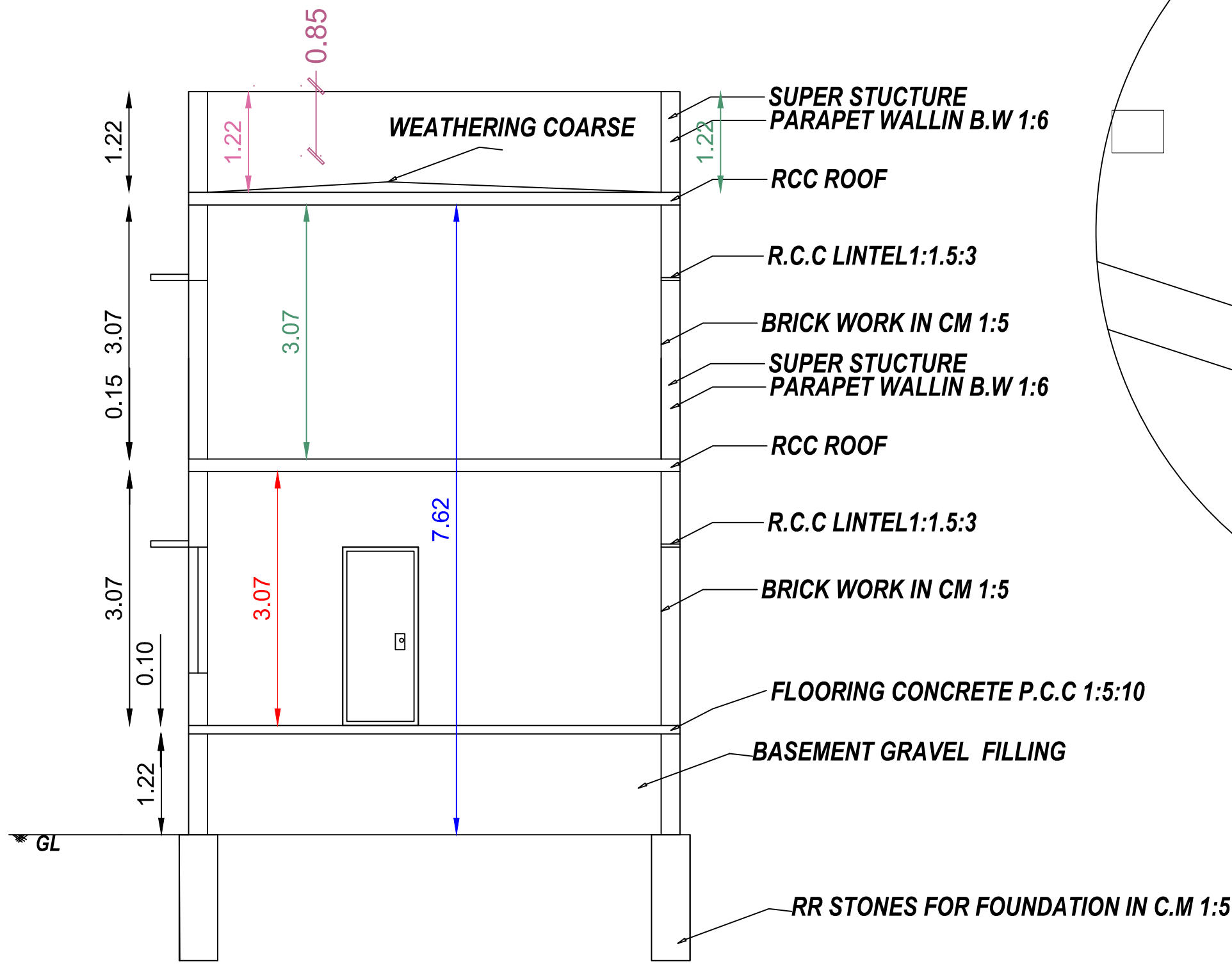
SECTION - A-A1
