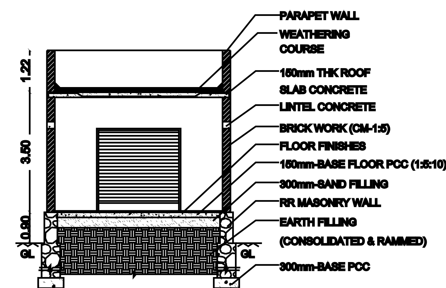
SECTION A-A
