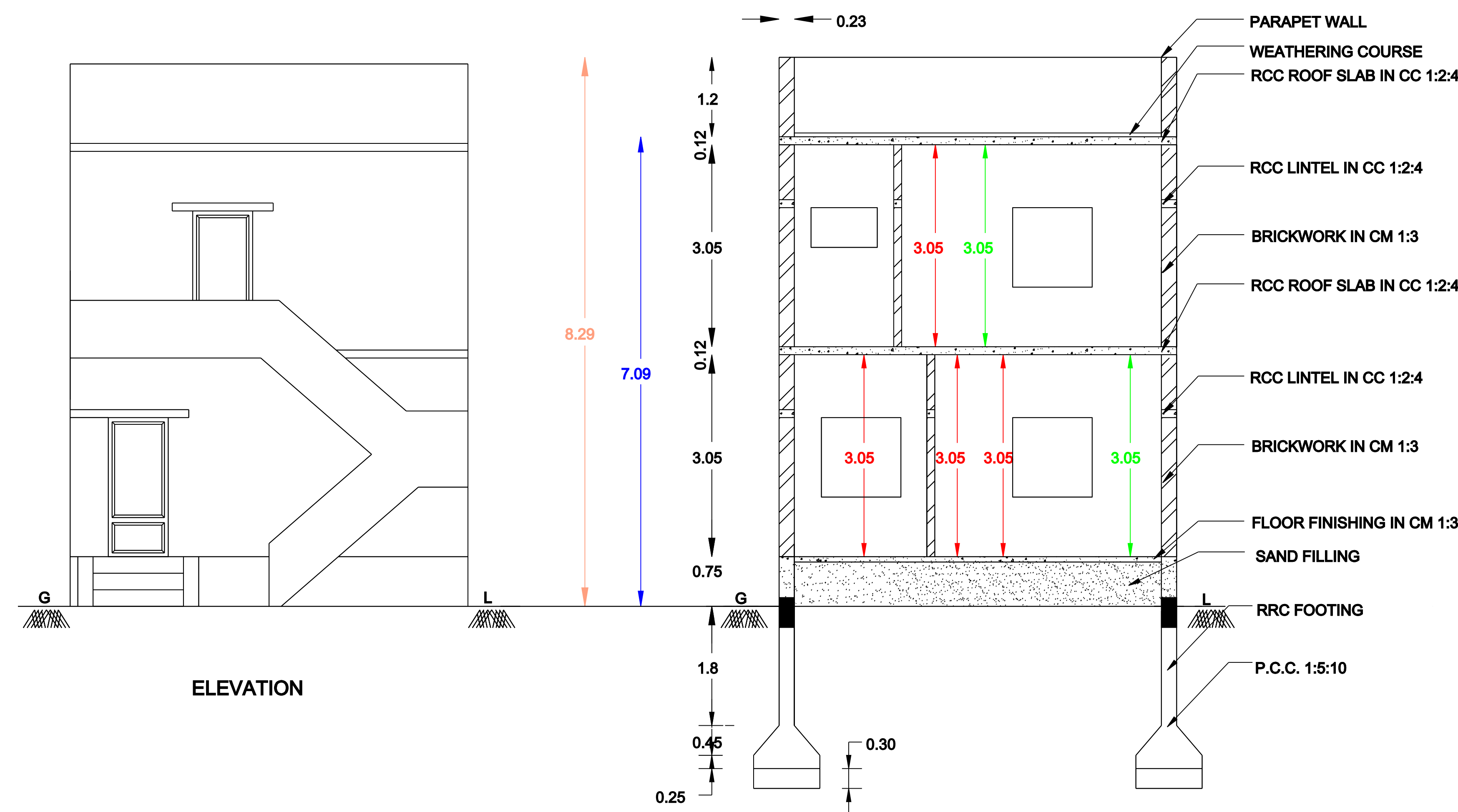
SECTION - AB
