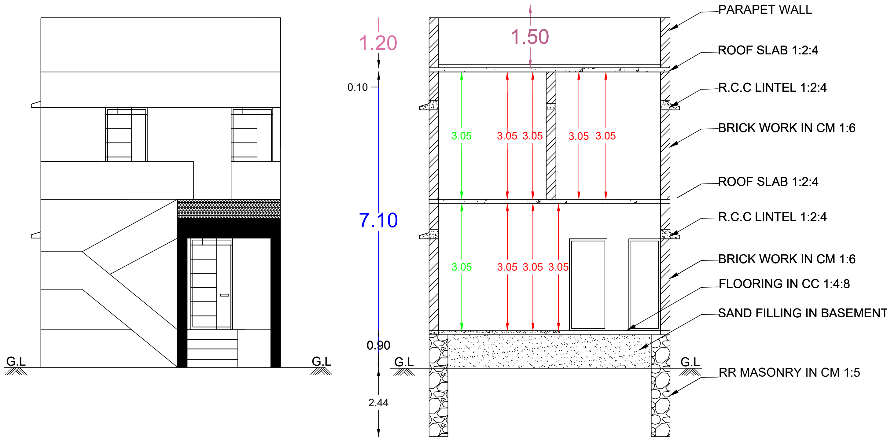
ELEVATION
