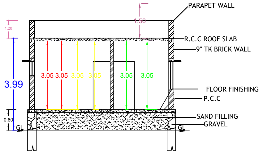
SECTION A-B
