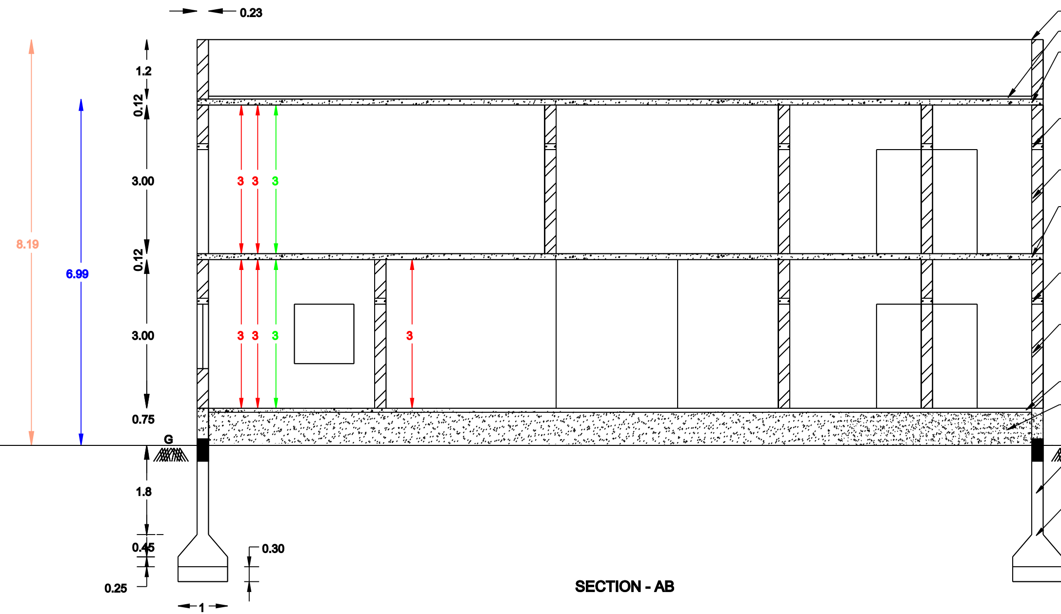
SECTION - AB
