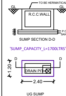
UG SUMP
