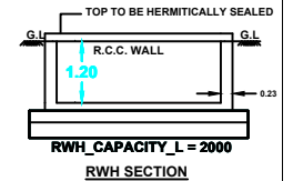
R.W.H. SECTION
