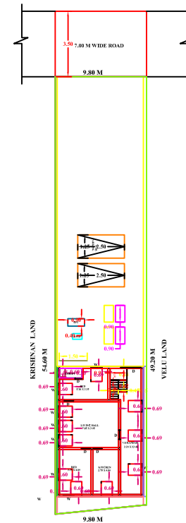
SITE PLAN SCALE : 1:200
