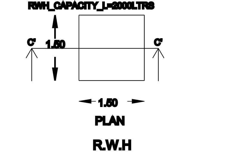
PLAN R.W.H
