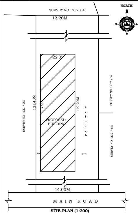
SITE PLAN (1:200)
