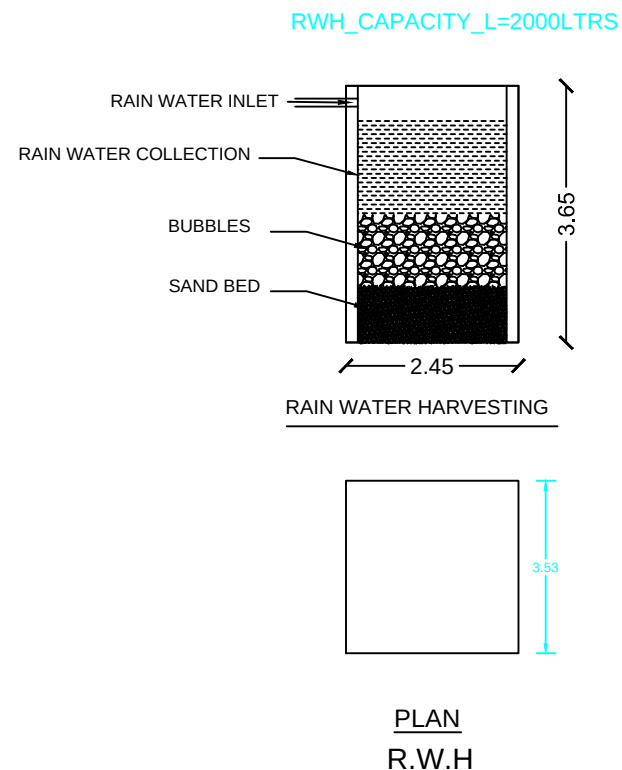
PLAN R.W.H
