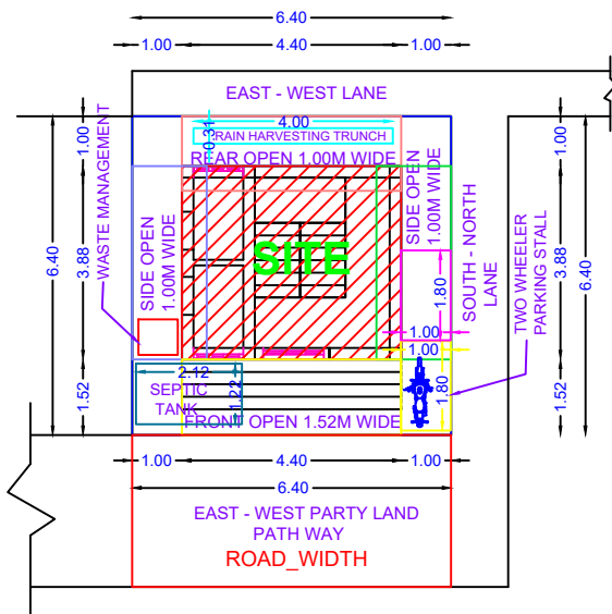
SITE PLAN SCALE 1:400
