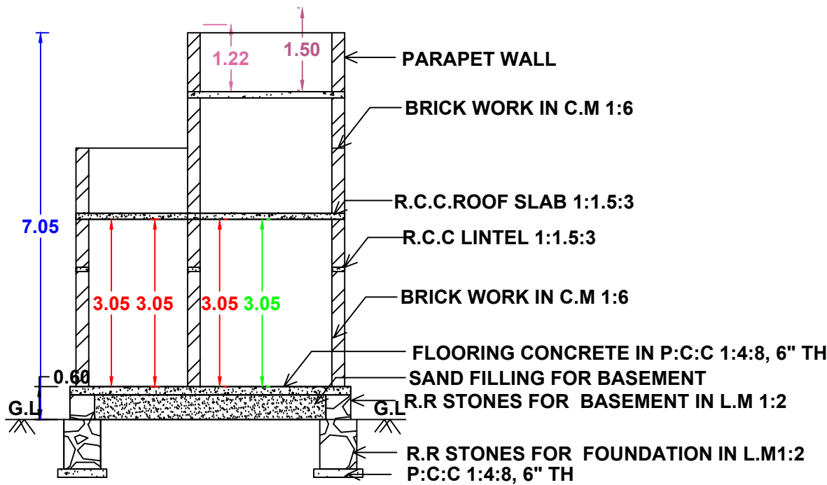
SECTION A-A
