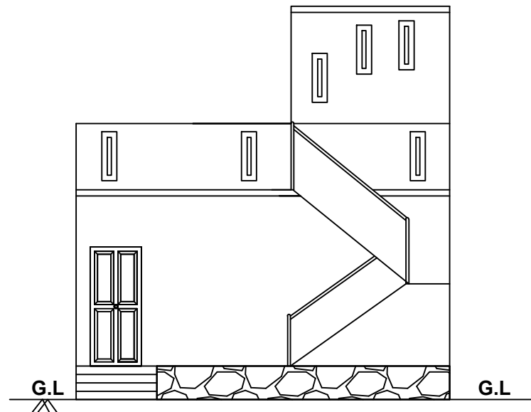
ELEVATION
