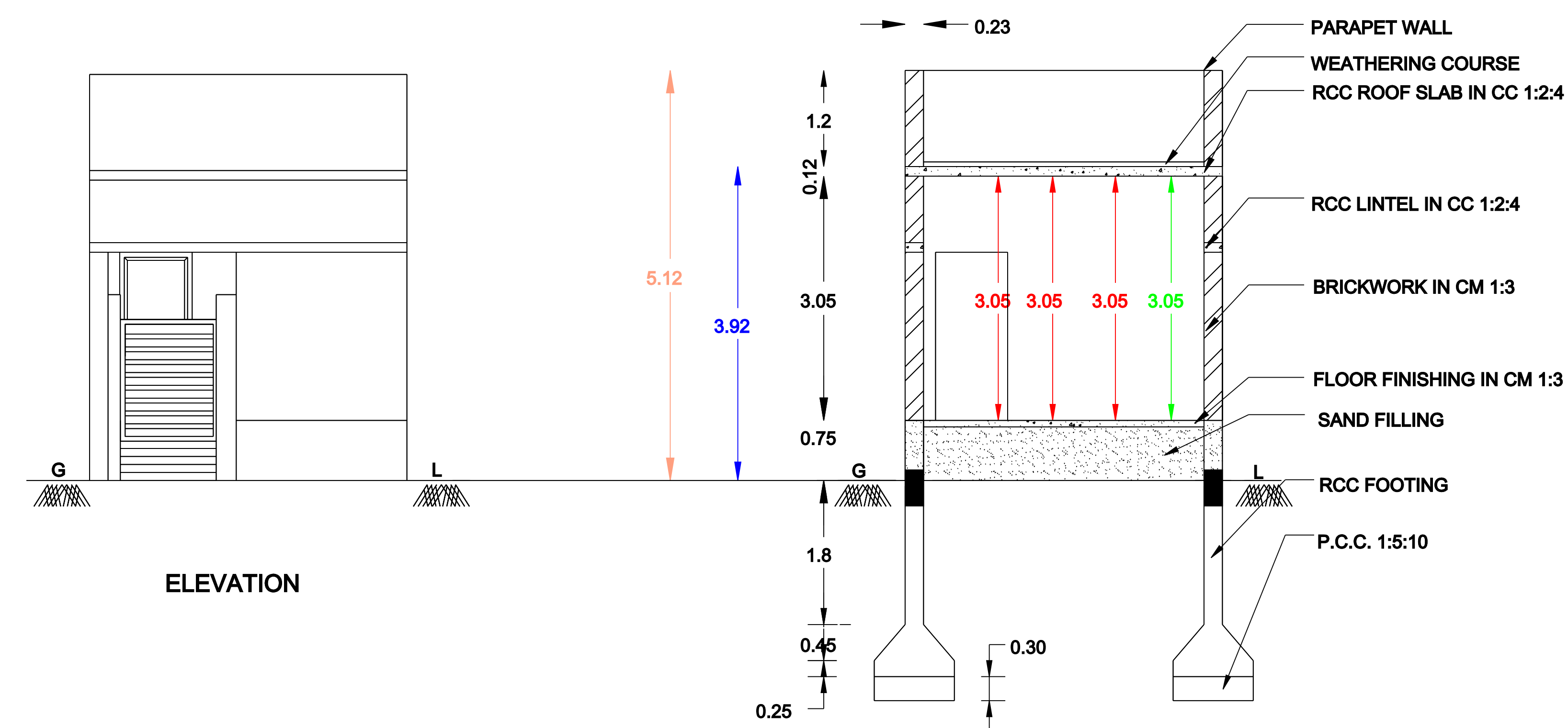
SECTION - AB
