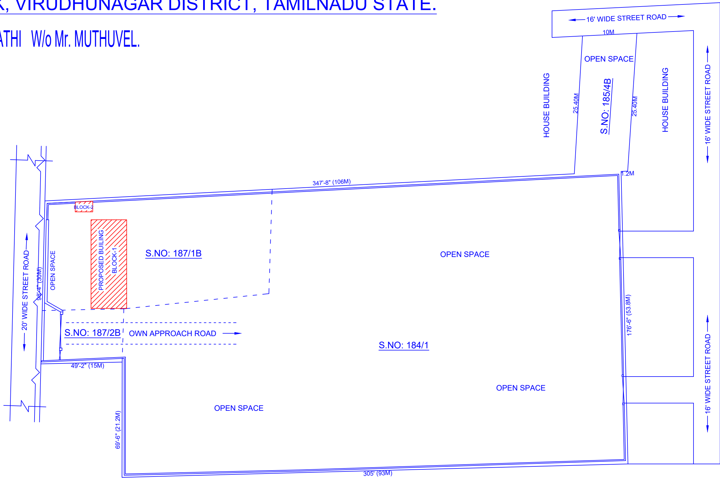
SITE PLAN SCALE 1 : 4M
