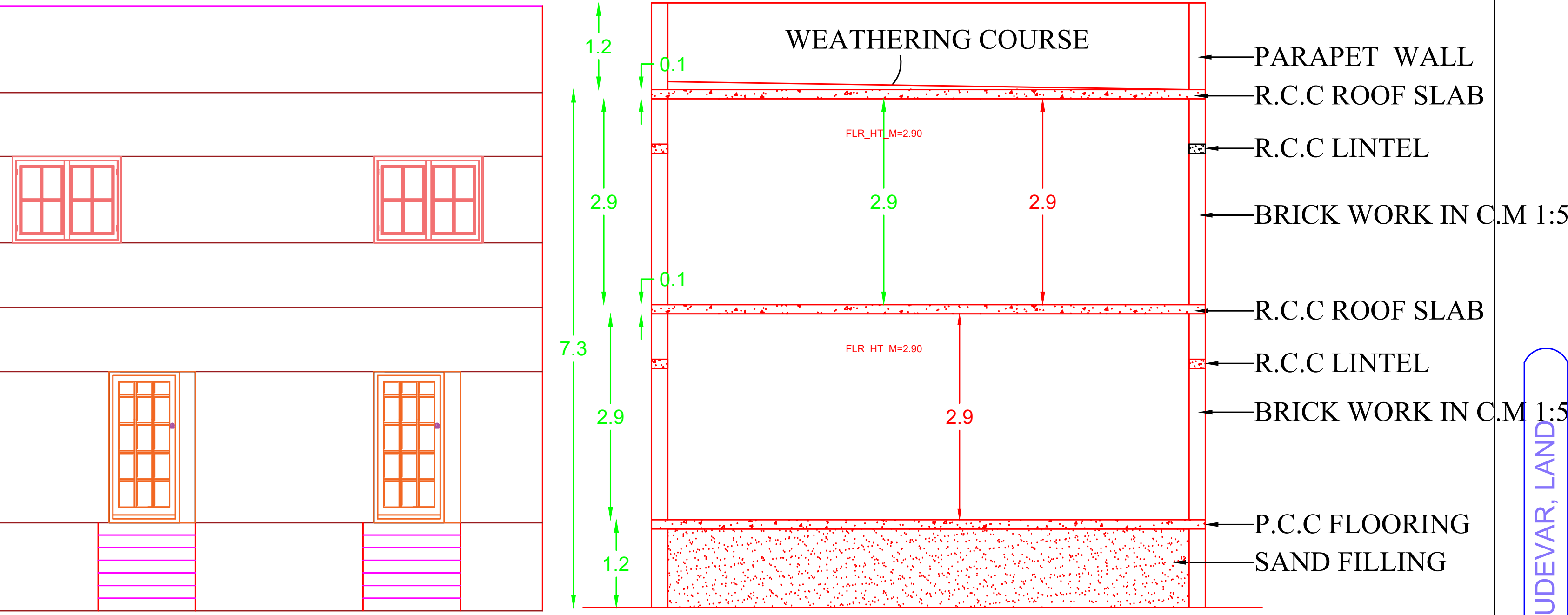
ELEVATION
