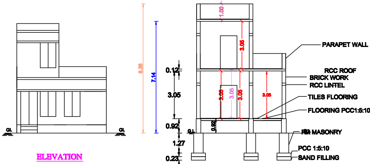
ELEVATION
