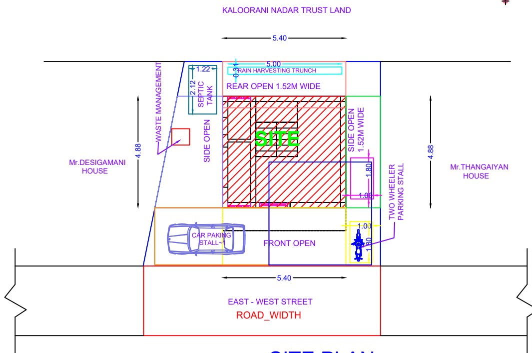
SITE PLAN SCALE 1:400
