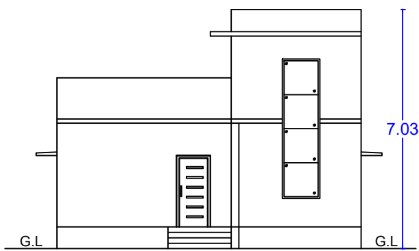
ELEVATION
