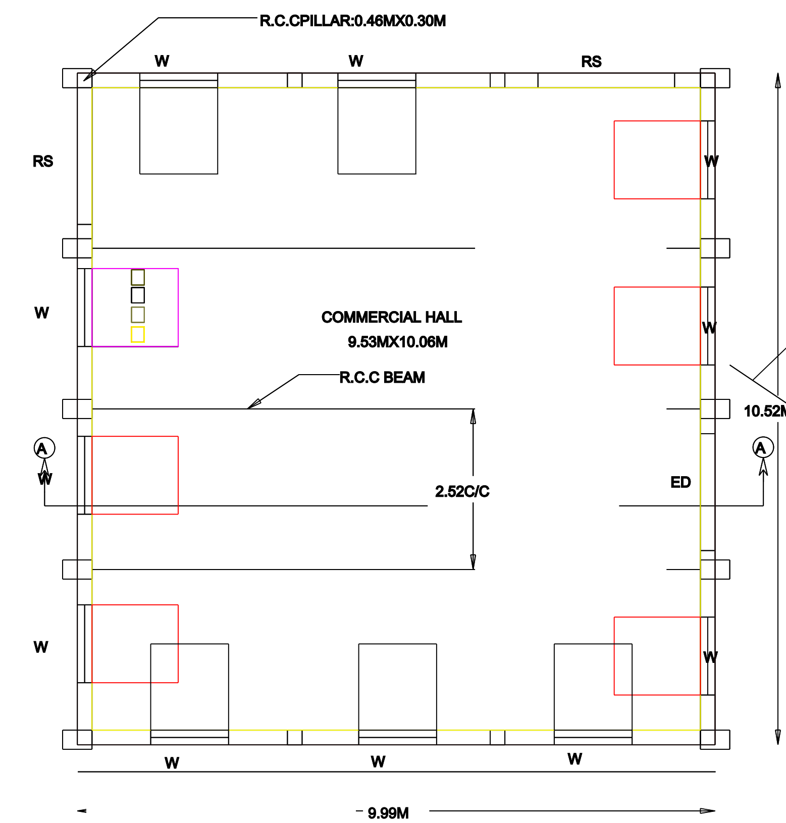
DOOR PLAN
