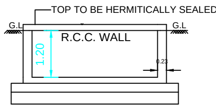
RWK SECTION ( SAMPLE) RWK_CAPACITY_L=2000
