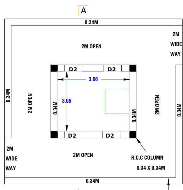
PLAN-2
