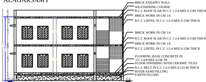
SECTION 'AB'
