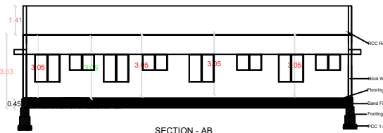
SECTION - AB
