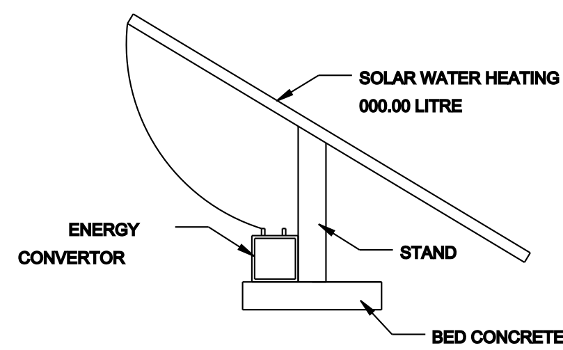
LONGITUDINAL SECTION
