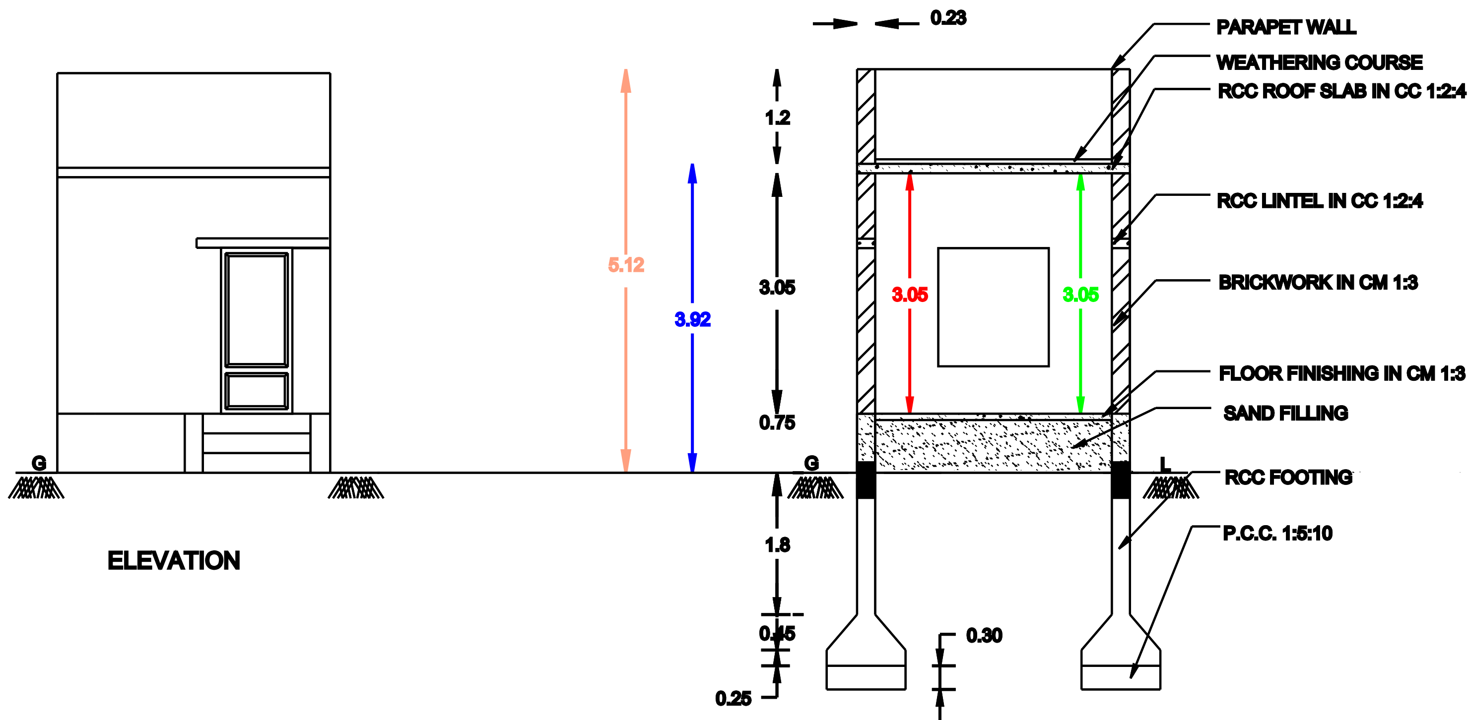
SECTION - AB
