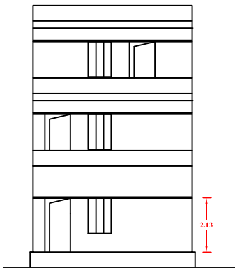
ELEVATION
