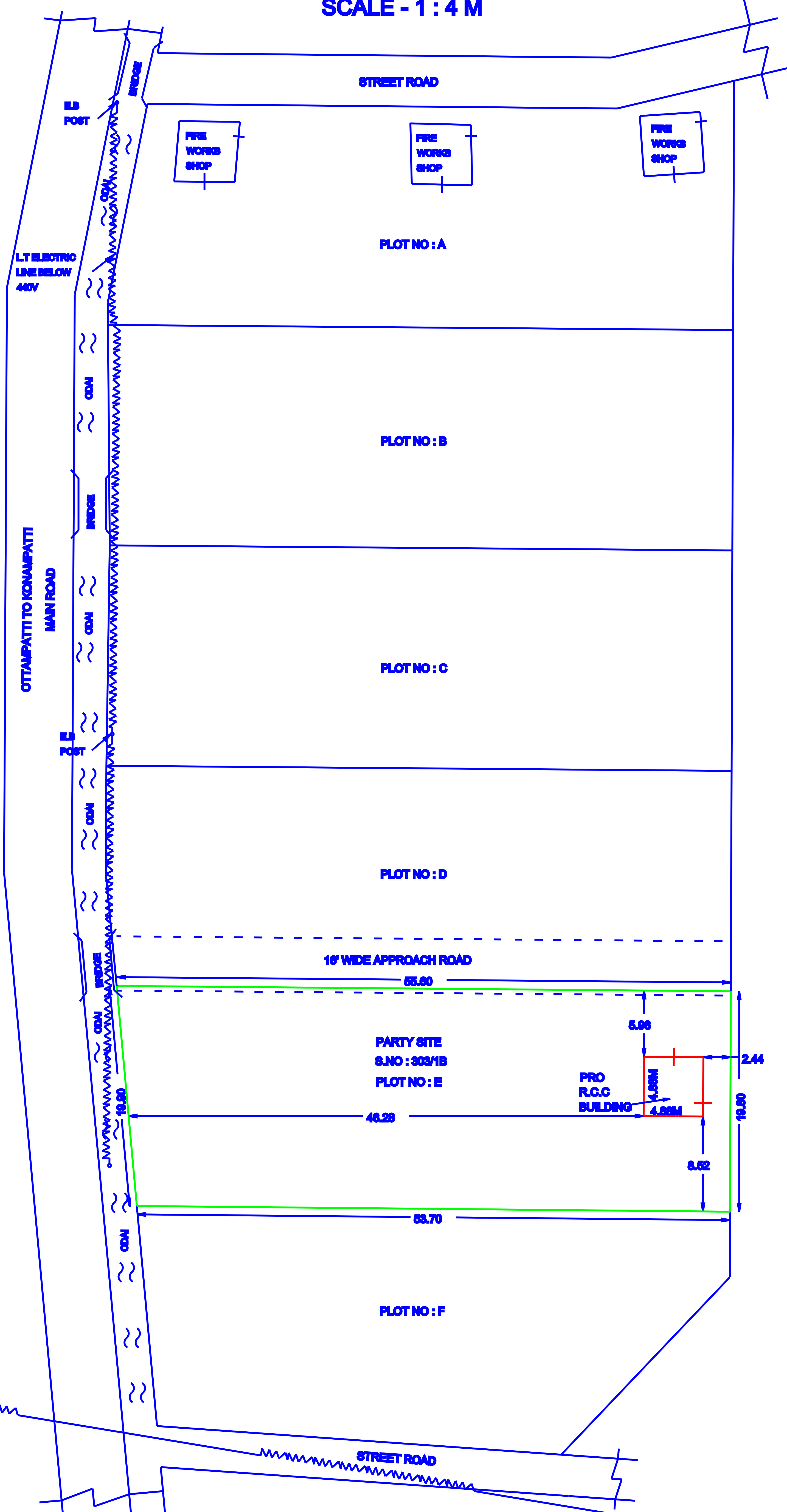
SITE PLAN SCALE - 1 : 4 M
