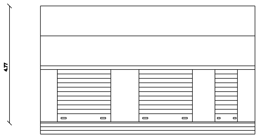
ELEVATION
