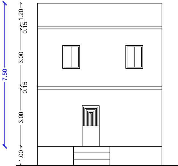
ELEVATION
