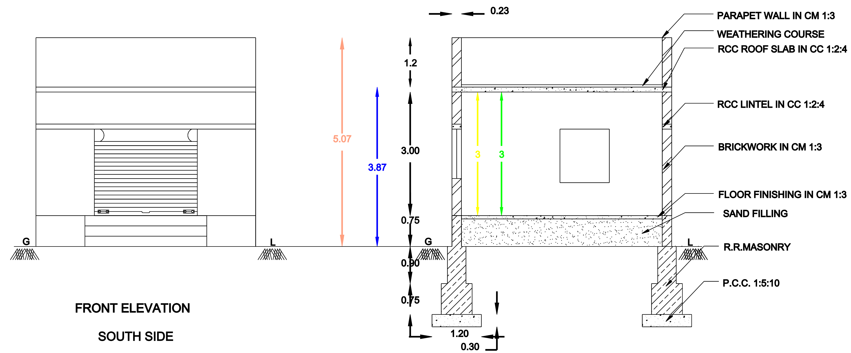
SECTION - AB
