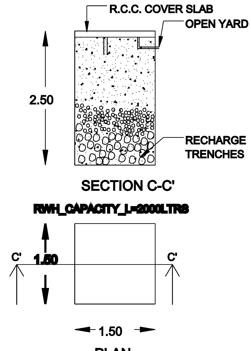
PLAN R.W.H
