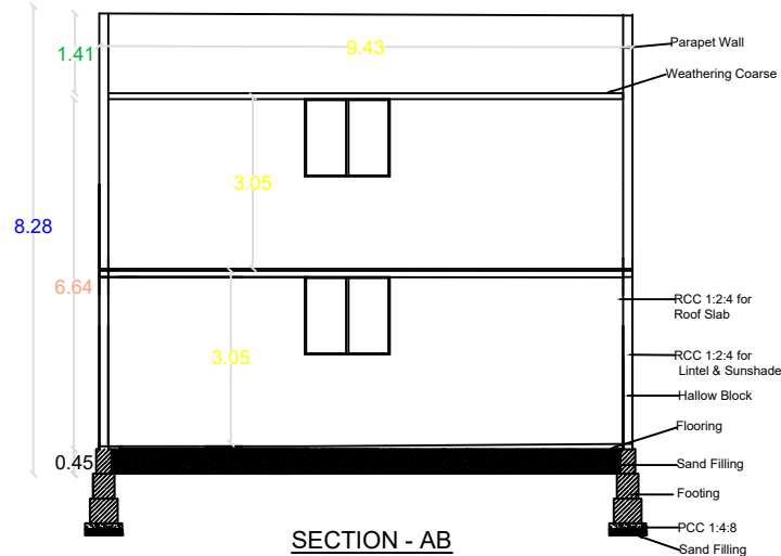
SECTION - AB
