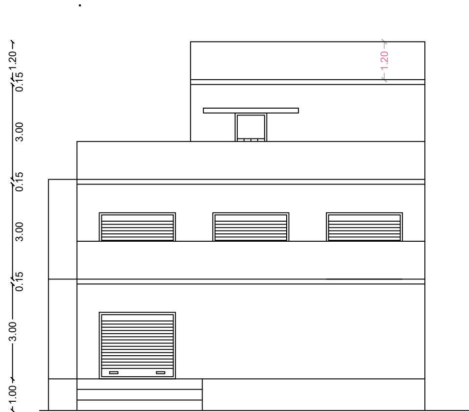
ELEVATION
