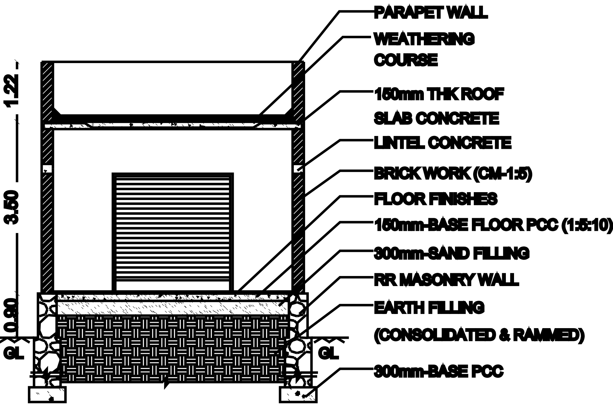
SECTION A-A
