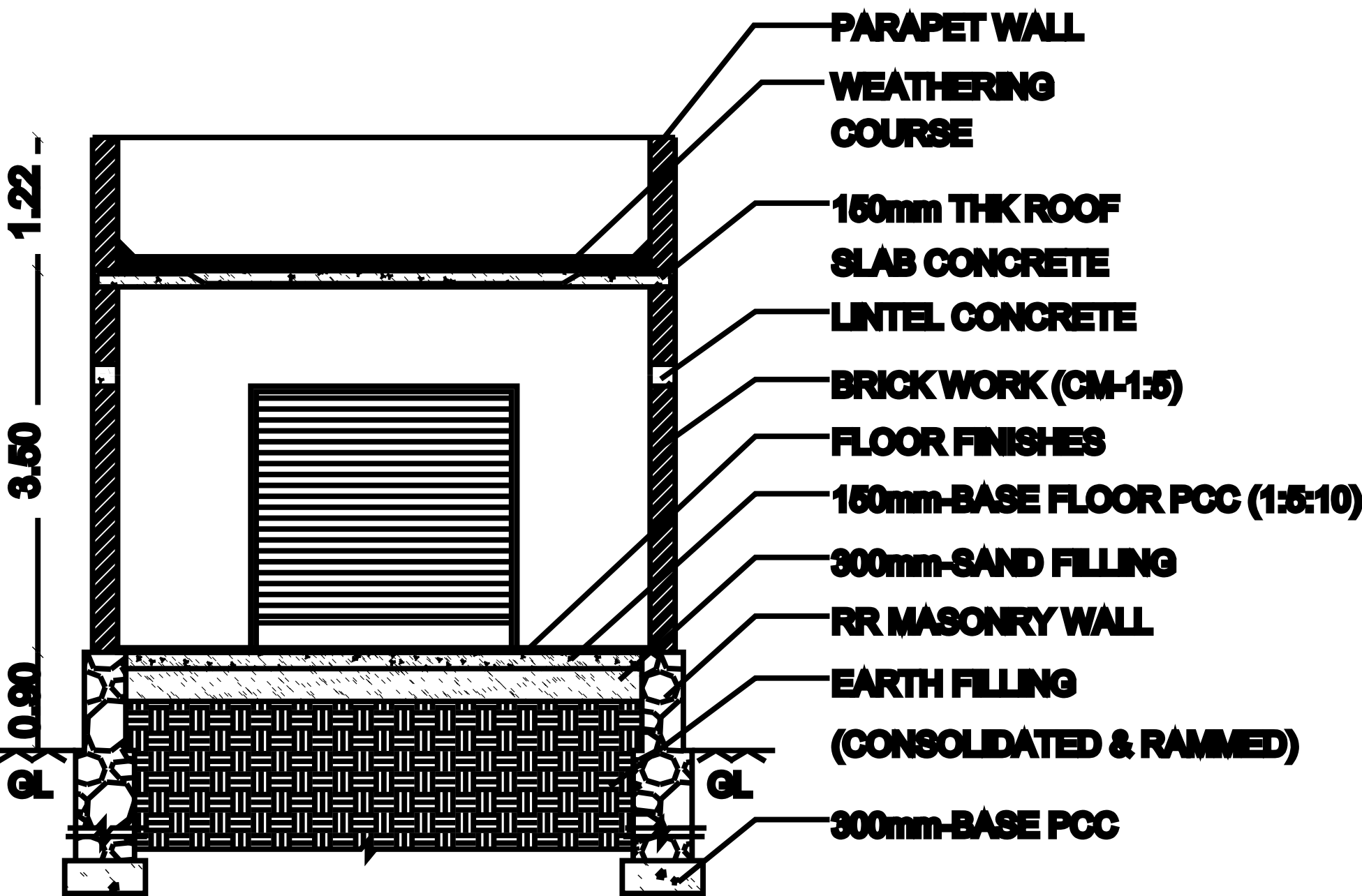
SECTION A-A
