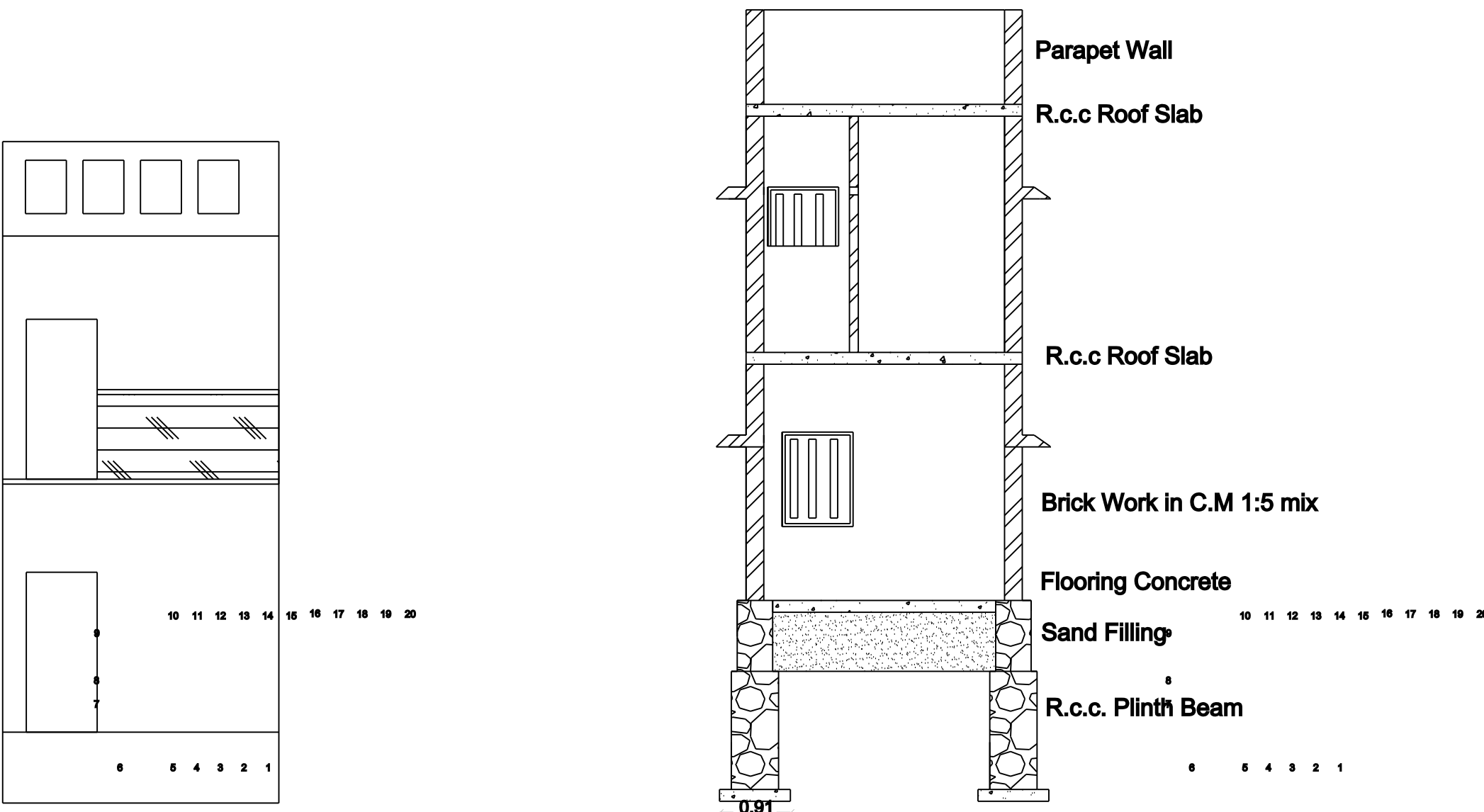
ELEVATION
