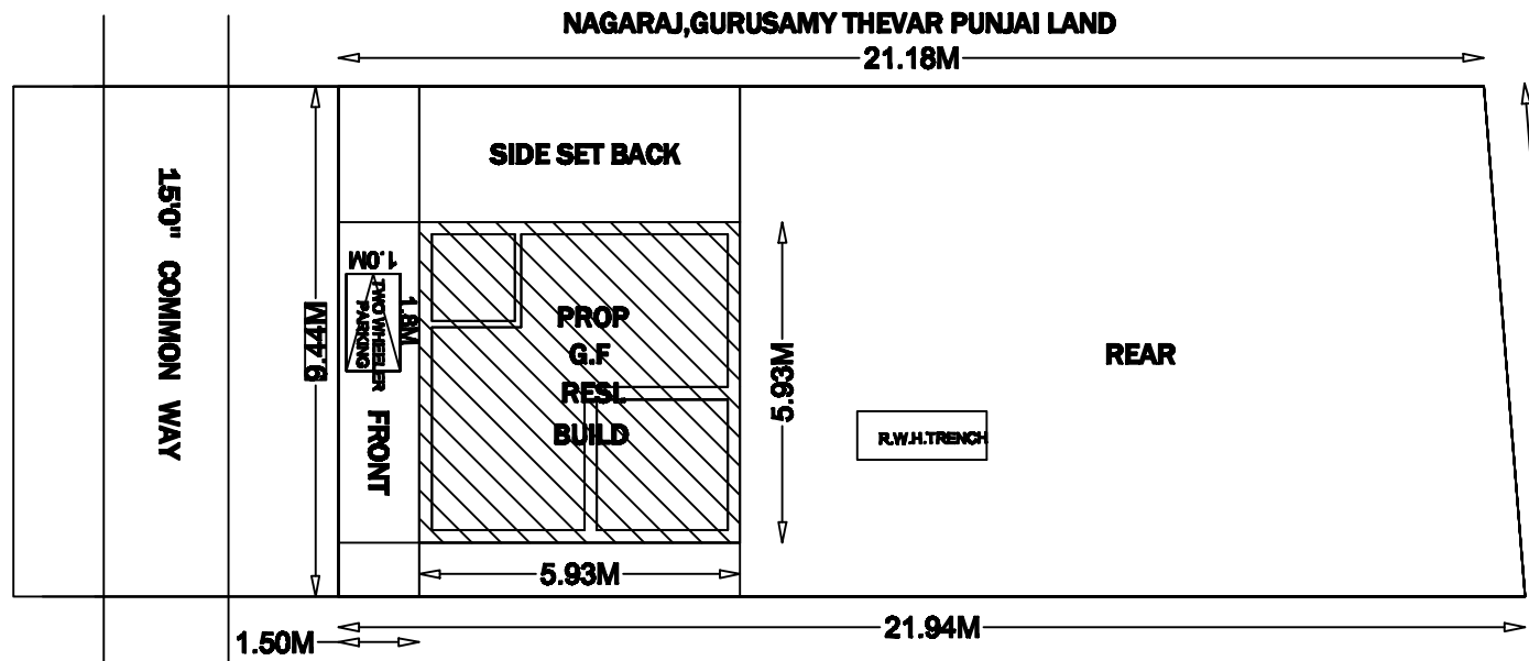
K.MARICHAMY LAND SITE PLAN, SCALE 1:100
