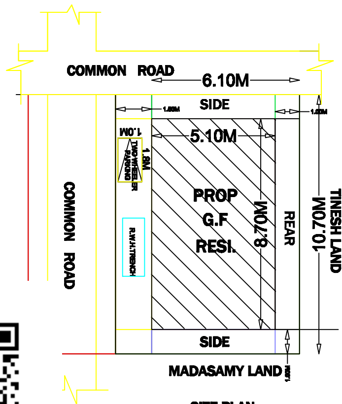
SITE PLAN, SCLAE 1:100
