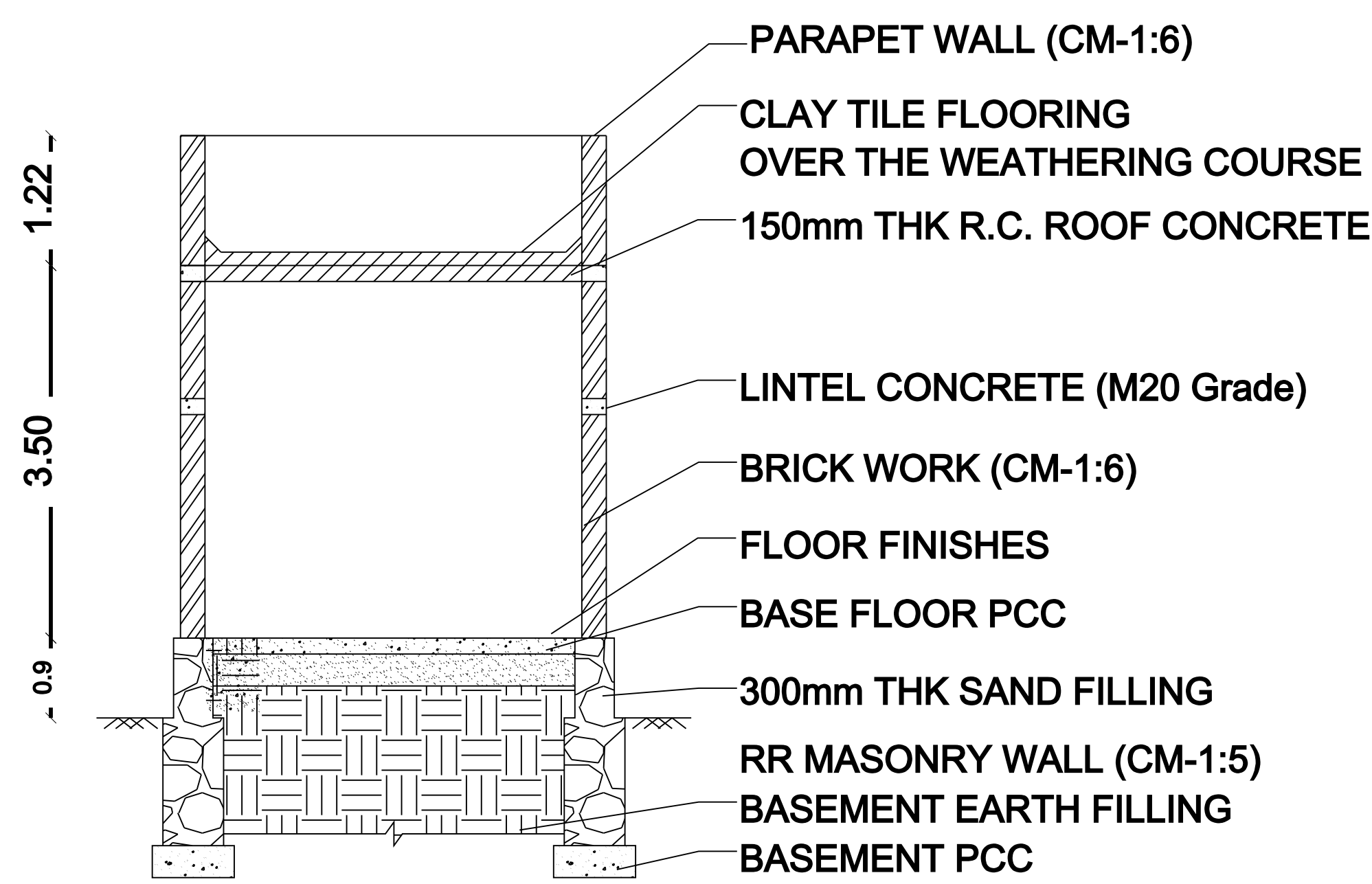
SECTION A-A
